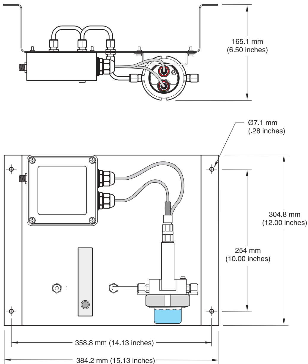
Figure 1 Dimension de Montage du Panneau
